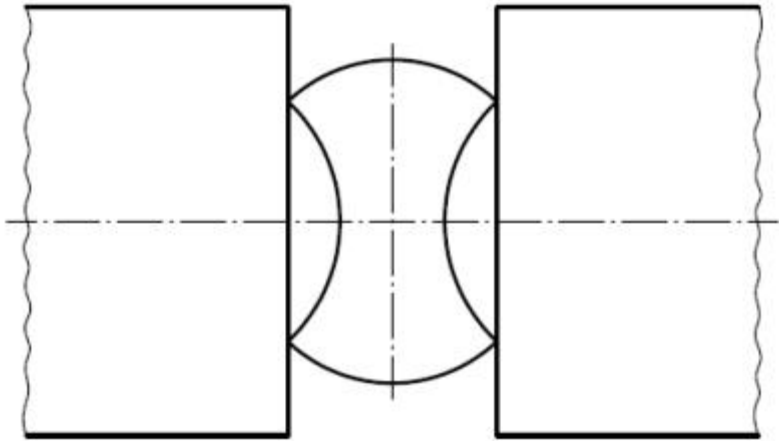
图 6 抗扭及抗弯性能试验中的夹持位置
