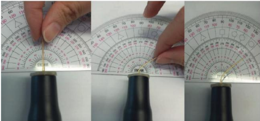
图 A. 6 用手将输送管弯曲到一个方向的 (45 \pm 5)^{\circ} 的示例
