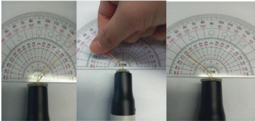
图 A. 7 用手将输送管弯曲到相反方向的 (45 \pm 5)^\circ 的示例
