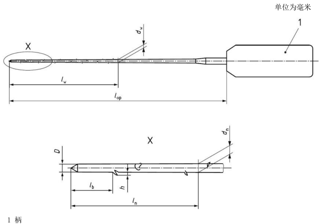
图 1 倒钩拔髓针-1 型辅助根管器械
