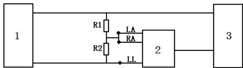
图中： 1—信号发生器 2—反搏装置 3—示波器 R1=100\text{ k}\Omega ，允差 \pm 0.1\% R2=100\text{ }\Omega ，允差 \pm 0.1\%
