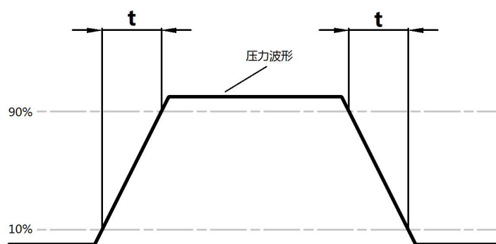
图 5 充排气过渡时间示意图
