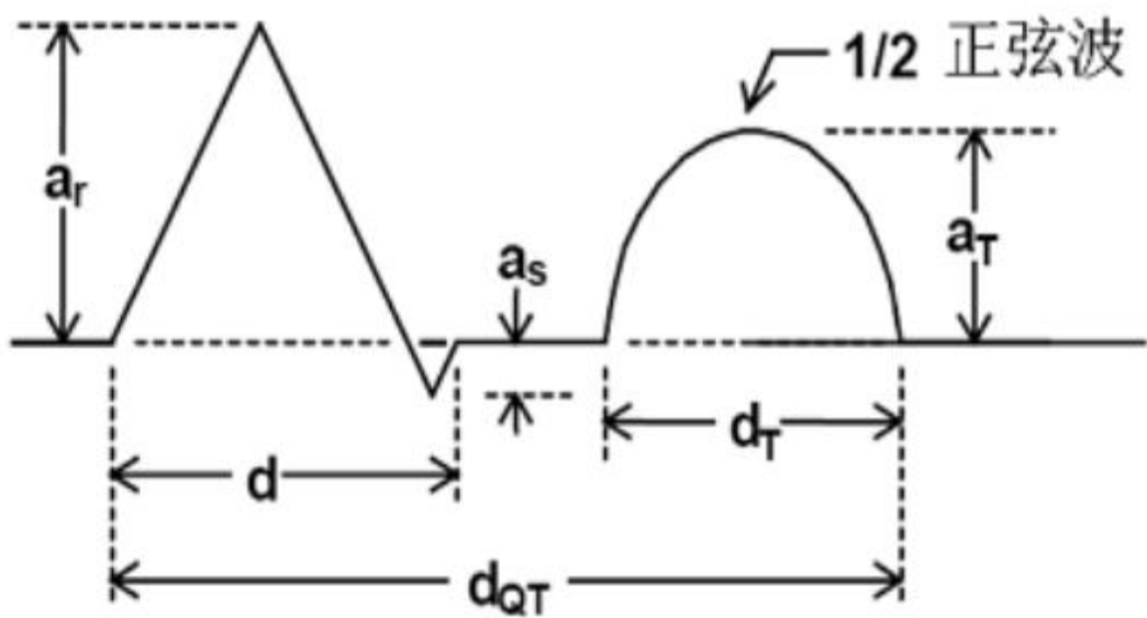
图 2 QRS-T 波
