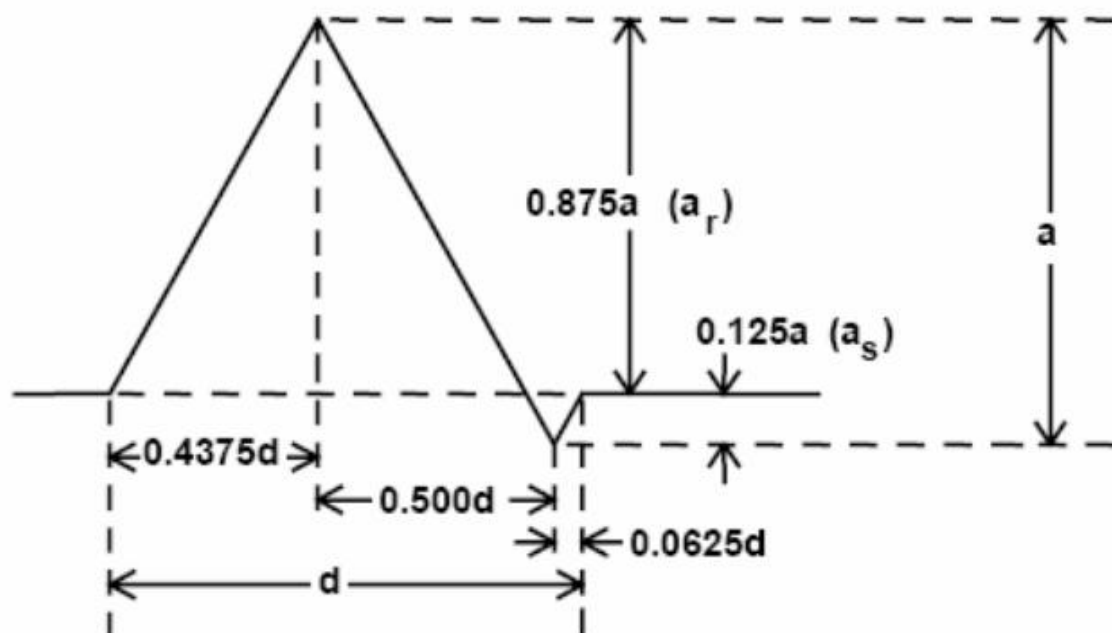
图 3 QRS 波
