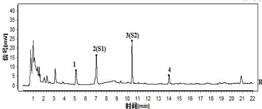
峰 2（S1）：鸟苷，峰 3（S2）：腺苷 冬瓜子配方颗粒对照特征图谱 色谱柱：HSS T3，2.1mm \times 100mm，1.8 \mu m
