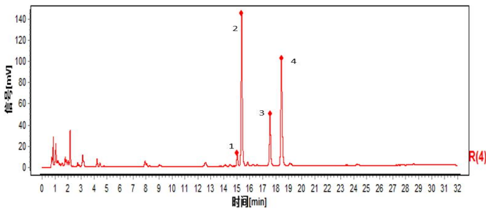
对照指纹图谱 参考色谱柱：Eclipse Plus C18 RRHD，2.1mm×100mm，1.8μm
